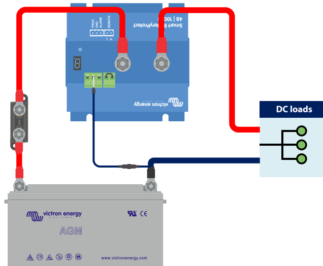
Smart BatteryProtect dans un système simple avec une boucle de fil entre les entrées L et H (réglage d'usine)
