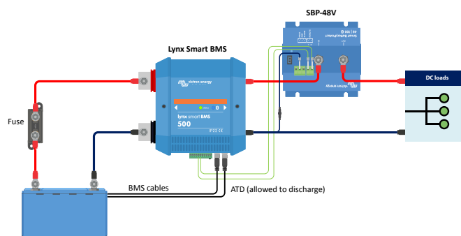
Smart BatteryProtect en mode lithium-ion contrôlé par ATD à partir d'un Lynx Smart BMS
