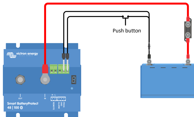
Bouton-poussoir câblé pour programmer le Smart BatteryProtect
