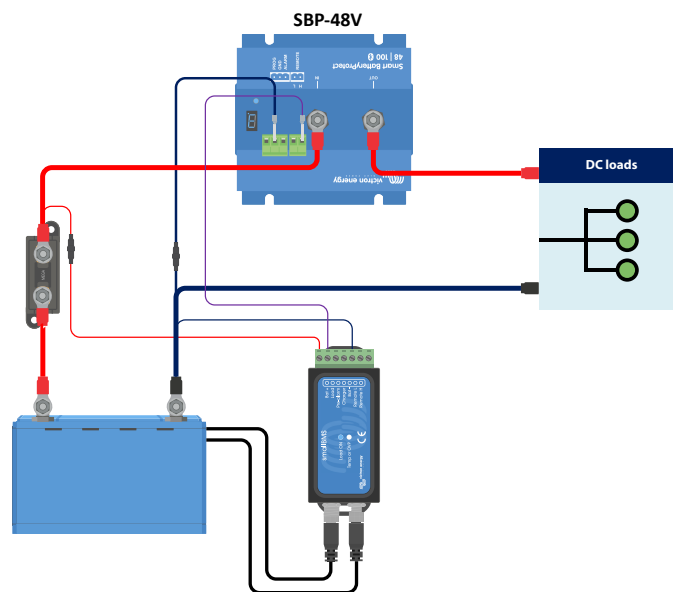
Le Smart BatteryProtect utilise la déconnexion de consommateur d'un smallBMS
